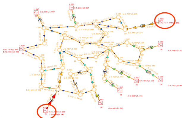
图 5-8 暂态稳定主导机组辨识
