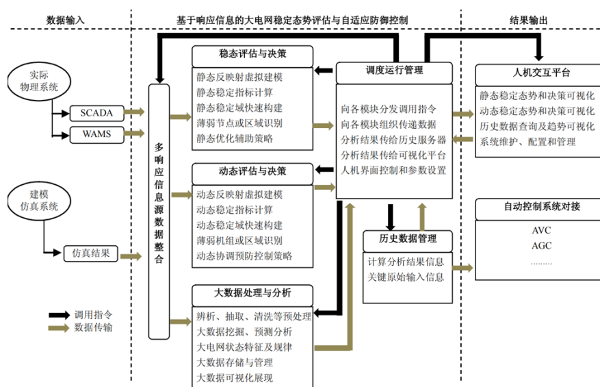
图 5-2 智慧电网调度软件架构
