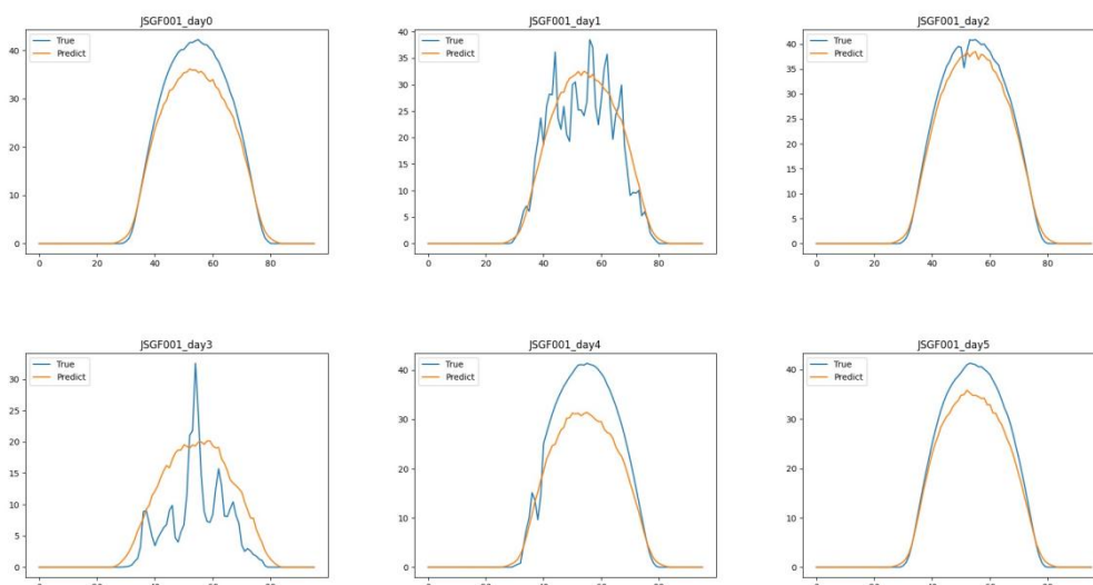
图 2-2 CNN-BiGRU 模型预测功率图
