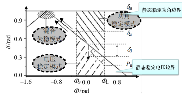
图 5-5 静态稳定运行域
