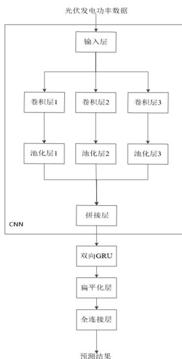
图 2-1 基于 CNN 和 BiGRU 的光伏发电功率预测模型结构图
