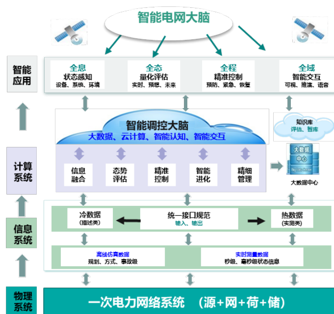
图 5-1 智慧电网调度功能架构
